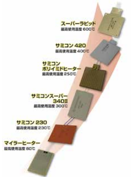
▲低温から高温まで取りそろえた面状ヒーターシリーズ
