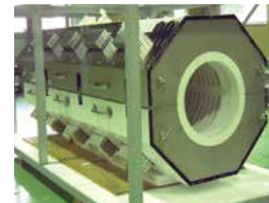
大型セラミックファイバー炉
